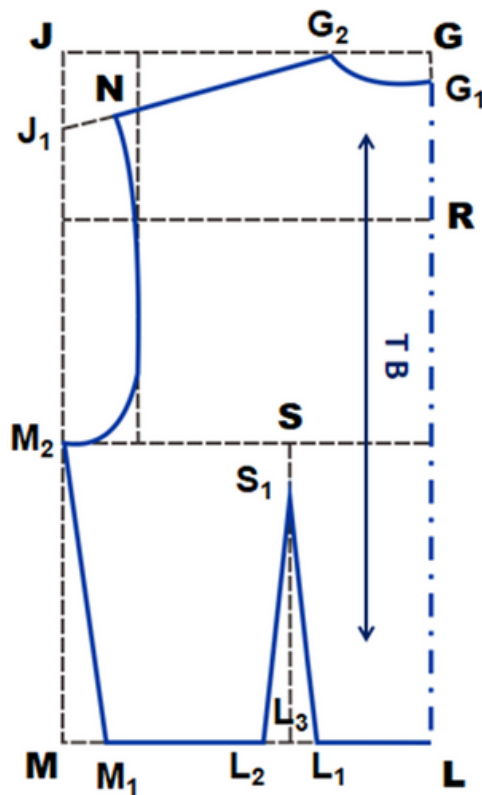
Gambar 2.10 Pola Dasar Badan Belakang dengan Sistem Praktis
